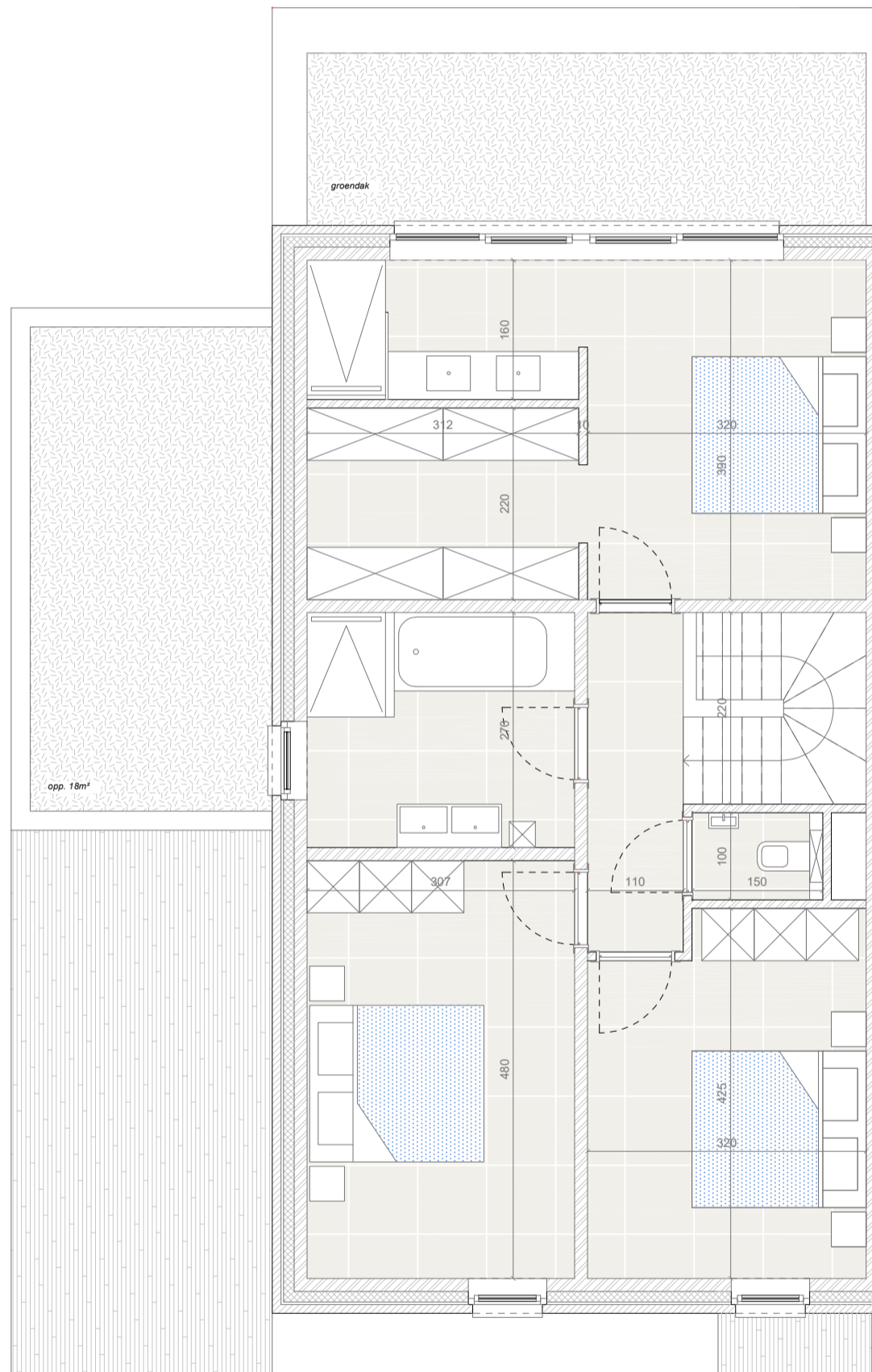
Woning 01 verdieping
