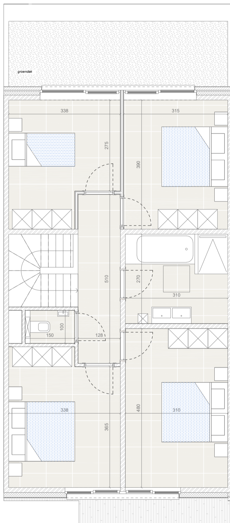
Woning 04 verdieping
