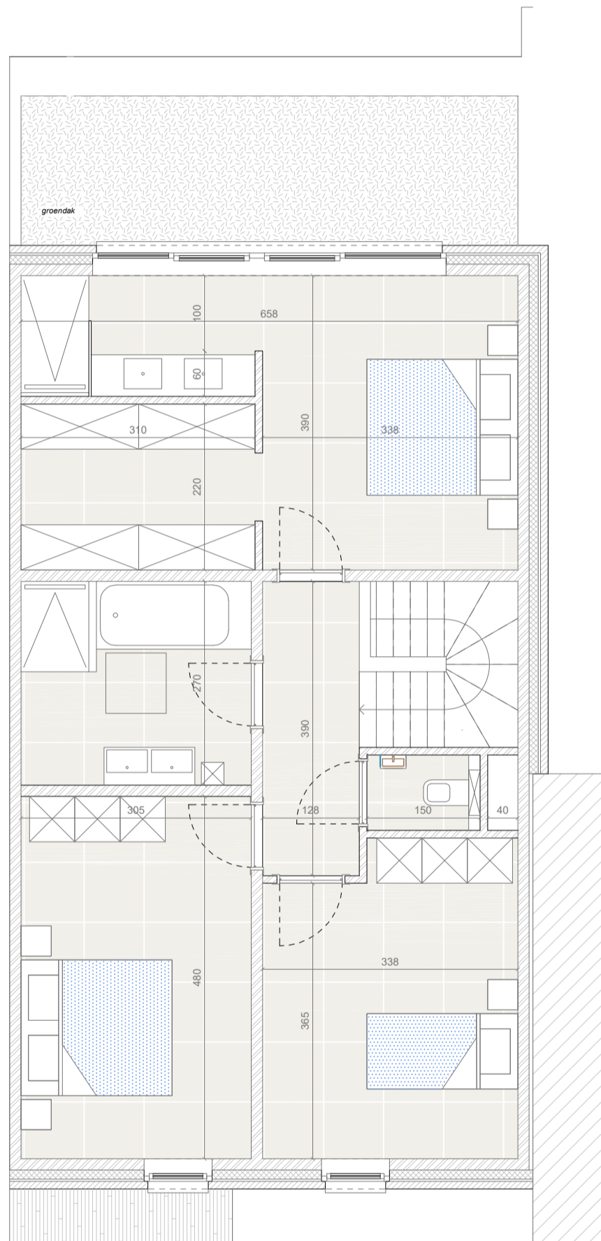
Woning 05 verdieping
